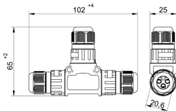
Conector estanco derivador
