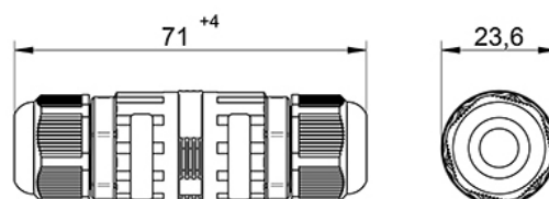
Conector estanco lineal
