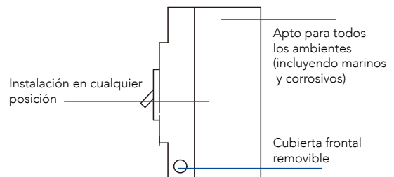
Interruptor caja moldeada de tipo fijo
