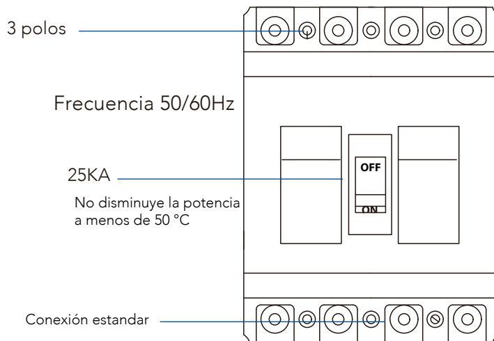
Interruptor caja moldeada de tipo fijo
